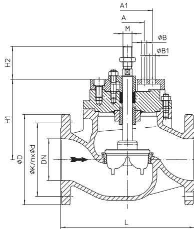
Fig. 470...90 DN200 (e.g.: DP34, PREMIO 5-15kN)
