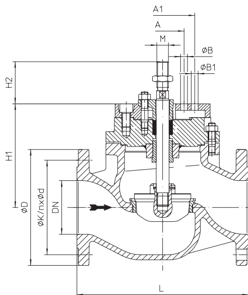
Fig. 470...90 DN150-200 (e.g.: DP34T-34Tri)
