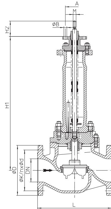
Fig. 471...90 DN200 M16 (e.g.: PREMIO 5-15kN, AUMA 07.6-10.2)
